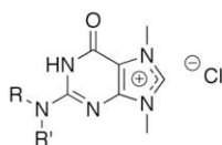
Heteromine D ( 1d ) R=R'=Me Heteromine E ( 1e ) R=Me, R'=H
