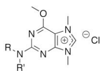
Heteromine A ( 1a ) R=R'=Me Heteromine B ( 1b ) R=Me, R'=H Heteromine C ( 1c ) R=R'=H
